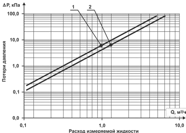
Рисунок 1 – Номограмма потери давления в теплосчётчиках
