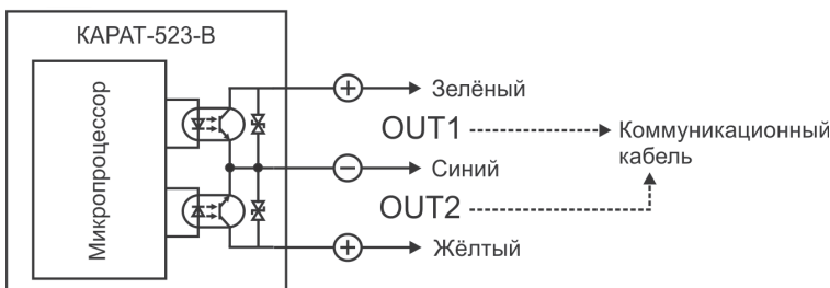
Рисунок 6 – Принципиальная схема подключения импульсных выходов
