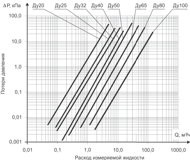
Рисунок 2 – Номограмма потерь давления для расходомеров
